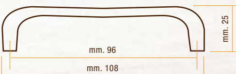
COD. 10.062 - COD. 10.162 con rondelle 41.062 COD. 10.262 con piastra 41.162
