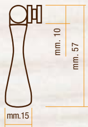
COD. 10.164 - COD. 10.264 con rondelle 41.062
