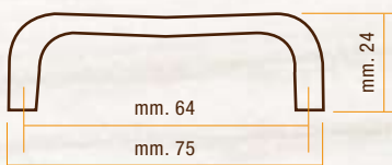
COD. 10.063 - COD. 10.163 con rondelle 41.063
