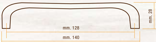
COD. 10.061 - COD. 10.161 con rondelle 41.062
