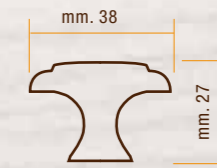
COD. 20.271 COD. 25.271 (zama)
